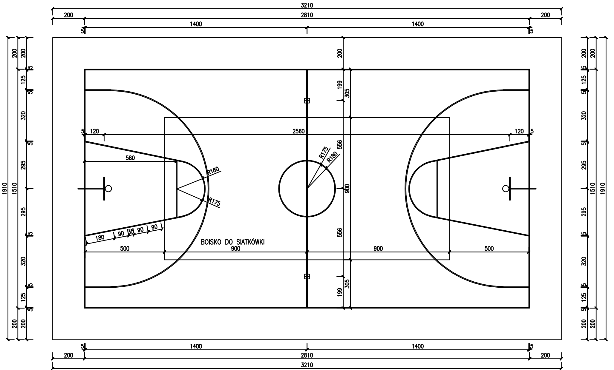
Boisko do koszykówki pełnowymiarowe Szerokość linii – 50mm, zalecany kolor czerwony
